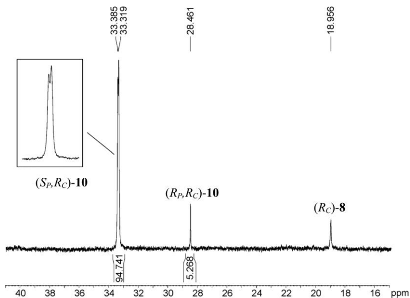
Figura 5. Espectro de RMN- ^{31}\text{P} (202.4 MHz) de 10 medido en THF- d_8 a -80 °C. Multiplicación exponencial de la FID (LB = 1) previa a la transformación de Fourier.
